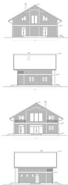
Фасады
