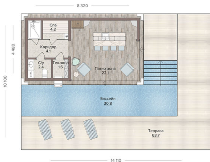
План 1 этажа
